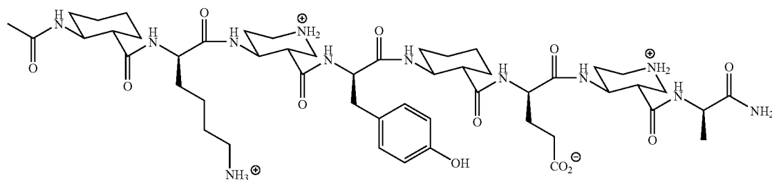
Ac-ACHC-K-PIP-Y-ACHC-E-PIP-A-NH 2 (SS) ACHC, (SS) PIP, (D) amino acids
