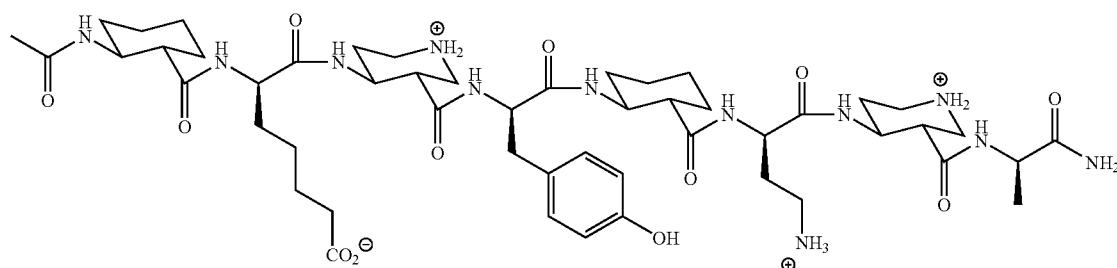
Ac-ACHC-E-PIP-Y-ACHC-K-PIP-A-NH 2 (SS) ACHC, (SS) PIP, (D) amino acids
