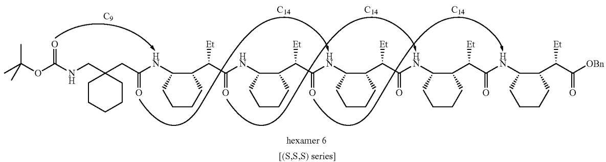
Scheme 7-7. Hexamer 6.
