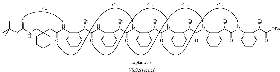
Scheme 7-8. Heptamer 7.
