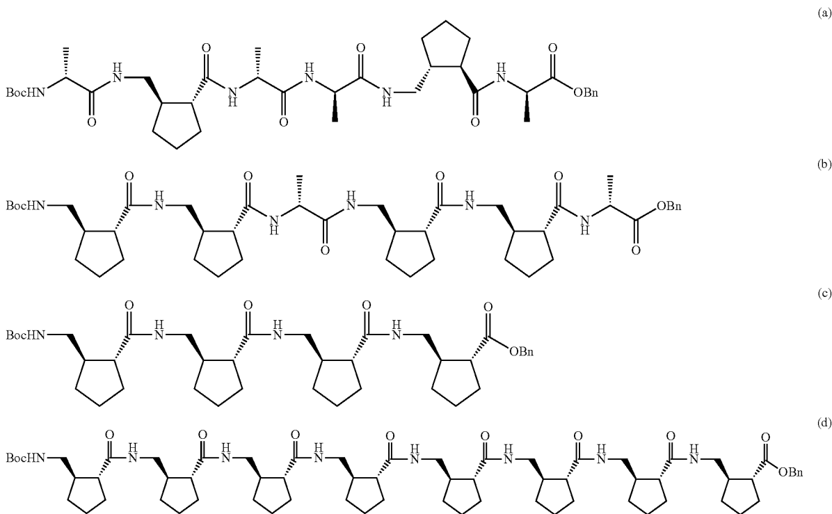
Scheme 5-6.
