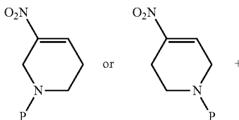
Scheme 3-2.
